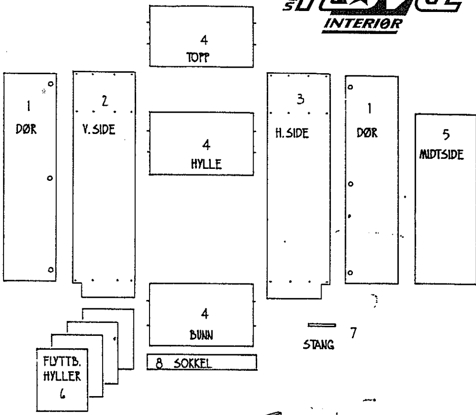
① SKROG MONTERES
