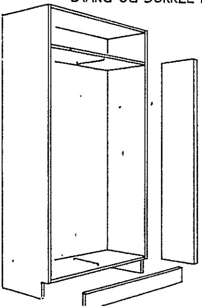
② MIDTSIDE OG HYLLER MONTERES STANG OG SOKKEL PÅSETTES
